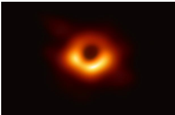
▲M87ブラックホール。強い引力で後ろ側のたくさんの星の光がねじまげられ、ドーナツ状に見える。(EHT Collaboration)
